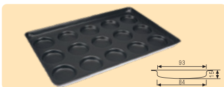
SN1613 0.8mm Alusteel 600x400x40mm | Ø93x84x15mm
